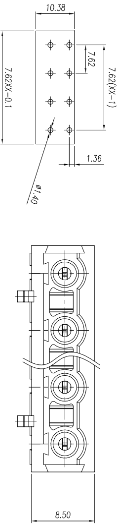
P.C.B. LAYOUT
